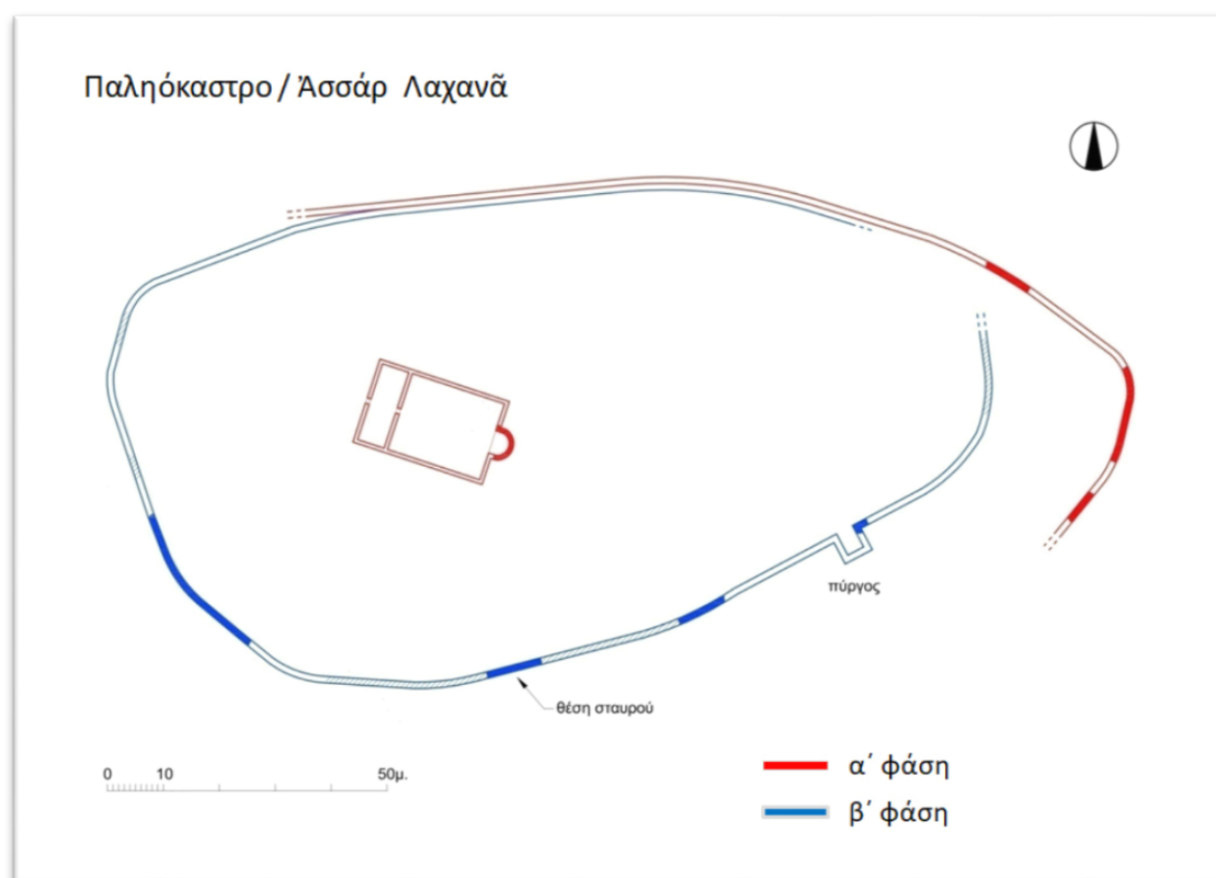
Εικ. 4. Παλαιόκαστρο / Ασσάρ Λαχανά. Οι δύο φάσεις της οχύρωσης (α' και β' φάση).
